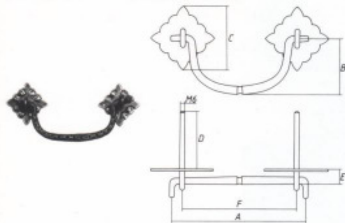
8613 Truhengriff Chest handle
