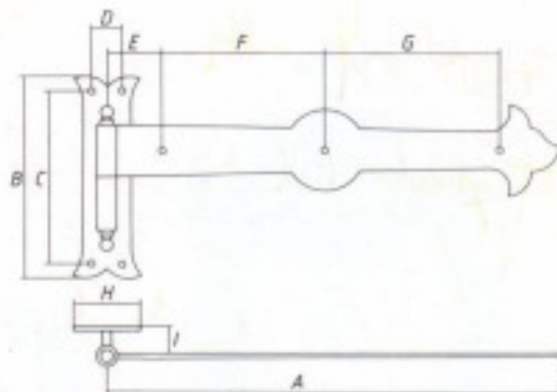
8669 Langband mit Kegel Hinge
