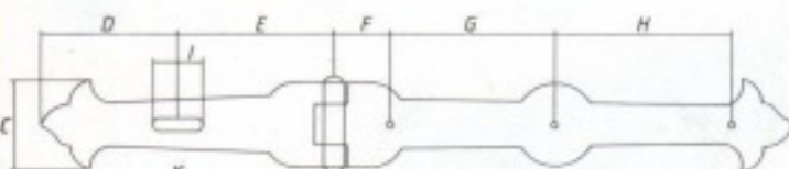
8614 Überfalle mit Schlaufe Chest hinge
